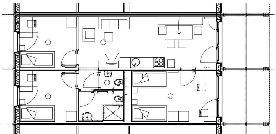
Wohneinheit 2 Module
