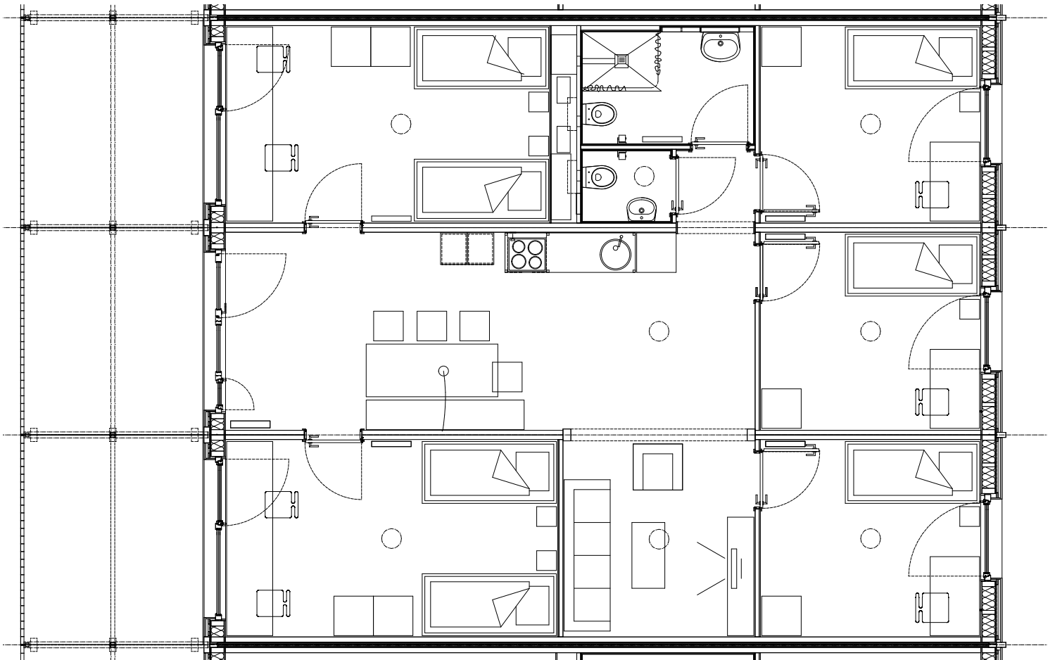
Wohneinheit 3 Module
